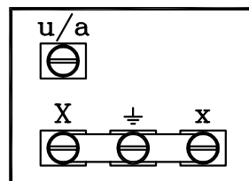
Klemmenbelegung bei einpoliger Ausführung
