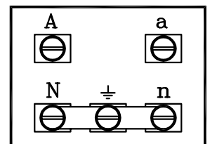
Klemmenbelegung bei einpoliger Ausführung mit en-Wicklung
